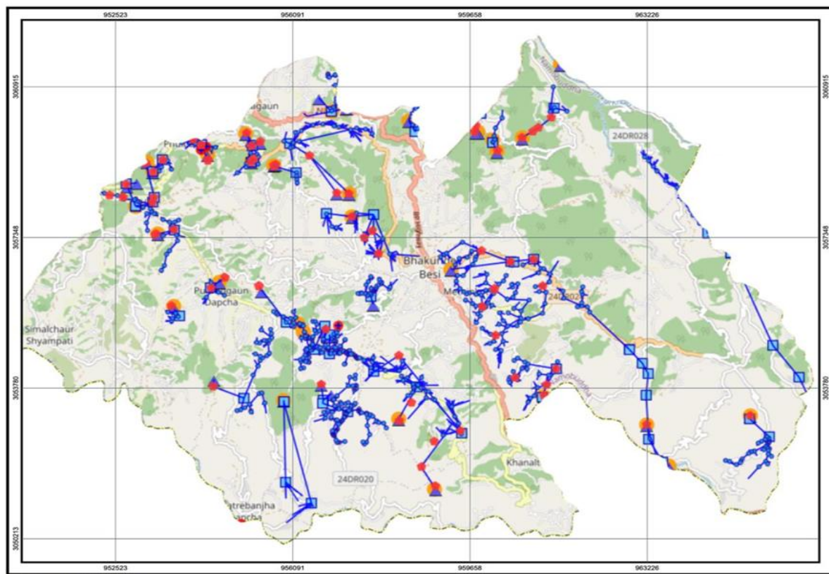
चित्र ११ : विद्यमान खानेपानी प्रणाली भित्रका योजना स्थान स्रोत
